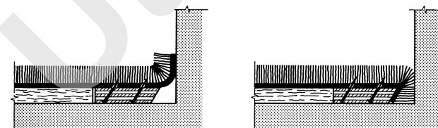
Fig. 53 d Teppekanten dyttes ned mellom pigglister og veggen.
