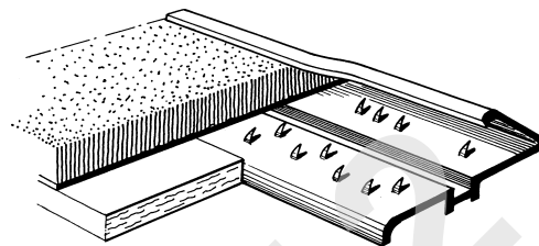
Fig. 55 a Eksempel på avslutning av teppe mot annet type belegg
