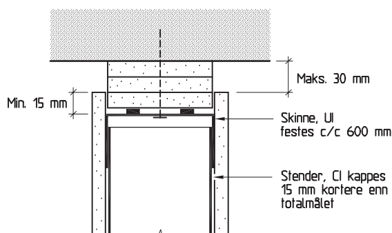
Fig. 83 Innervegg mot etasjeskiller av betong/lettbetong – teleskopløsning Løsningen gir normalt luftlydisolasjon R'_w = 37-40 dB, avhengig av flankeoverføringsbidraget via etasjeskiller.
