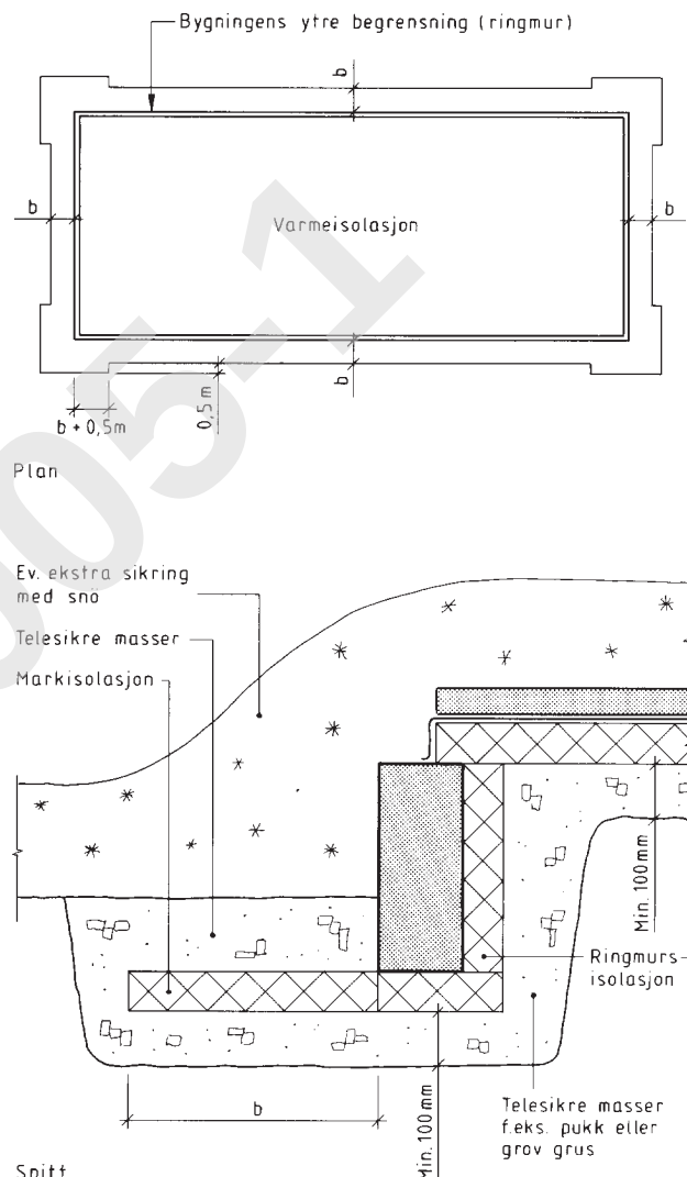
Fig. 24 a Frostsikring av golv og ringmur med varmeisolasjon
