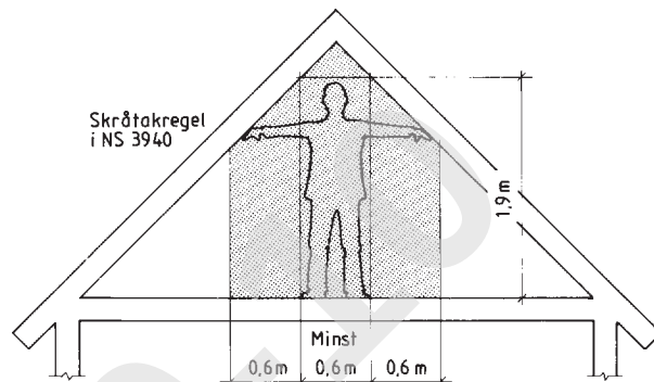
Fig. 11 Måleverdighet. For å være måleverdige, må rom (eller del av bygning) være tilgjengelig via dør eller trapp, fast eller nedfellbar. Det må ha golv og en takhøyde på min. 1,9 m i en bredde av 0,6 m. Under skråtak regnes areal som måleverdig til 0,6 m utenfor høyden på 1,9 m. På figuren er bruttoareal, bruksareal og nettoareal like store.
