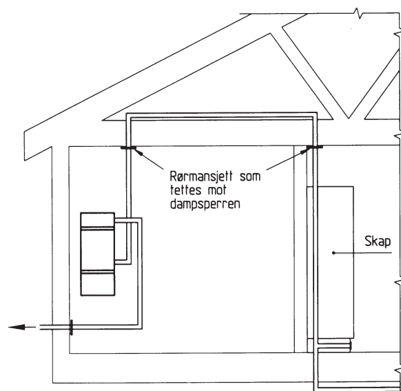
Fig. 37 Eksempler på rørføring ved installering av sentralstøvsugeranlegg i eksisterende hus
