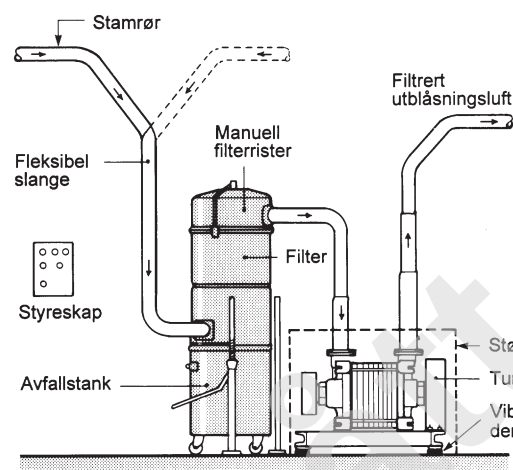
Fig. 61 b Støvsugersentral av større type for inntil åtte samtidige brukere. Plassbehovet er ca. 1,5 m x 2 m golvareal. Ved å parallellkoble flere støvsugersentraler kan antall samtidige brukere doubles, tredobles osv.
